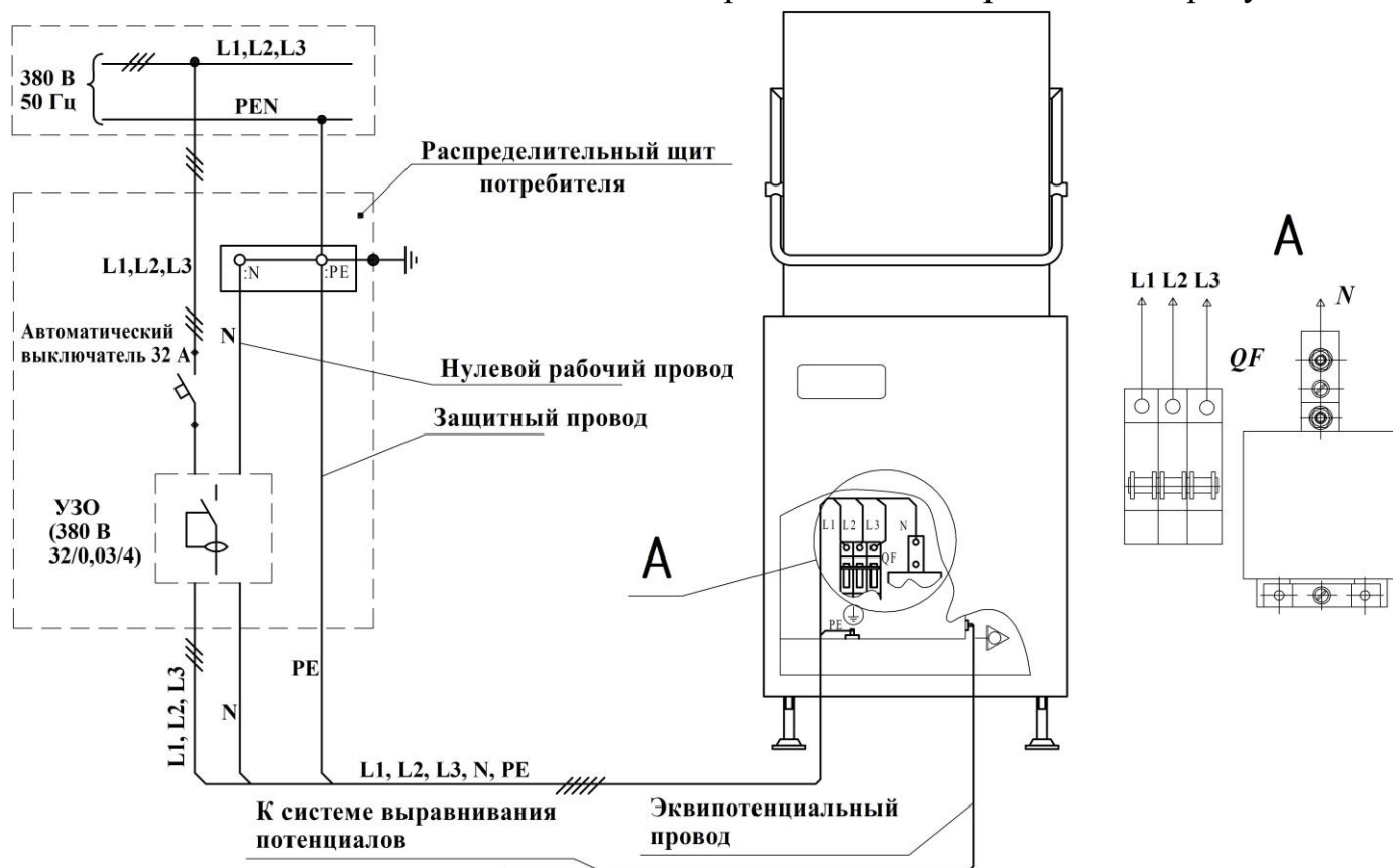
Рисунок 8 – Схема подключения машины к электрической сети
